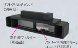
リフトグリルチャンバーは 背面(吸込口側)に取付けます。
